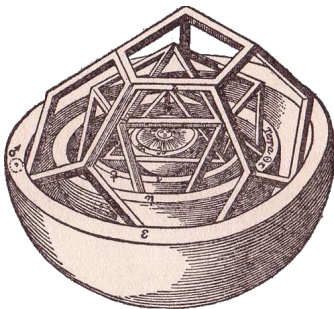
Le cosmographe de Kepler
